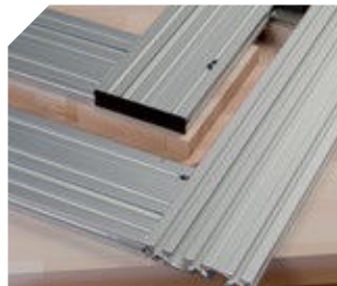
Equipada con accesorio para encajes rectos (sin radio), evitando el posterior relleno con masilla.
