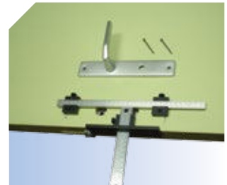
Taladrado de accesorios para puertas.
