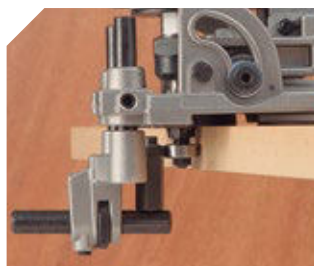
Freno del rodamiento de la fresa para evitar marcas sobre el panel.
