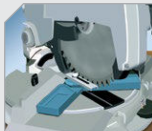
Con la sierra paralela al ángulo indicado por la guía de corte, se consigue un inglete exacto
