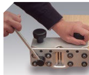
Corte sin esfuerzo de manera precisa y estable gracias a la palanca de corte y sus dos pomos de sujeción.
