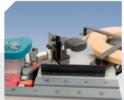
5046266 Cjto cortador + portarrollos RC50T (para MEB250, MEB100)
