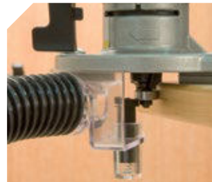
Conexión para la aspiración dotada de un freno para el rodamiento, que evita marcar el canto.
