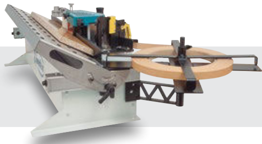
5046703 Perfilador AK97NW + prensos + rodillo (para MEB250, MEB250A)
