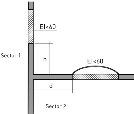
Figura 2.1. Encuentro cubierta-fachada
