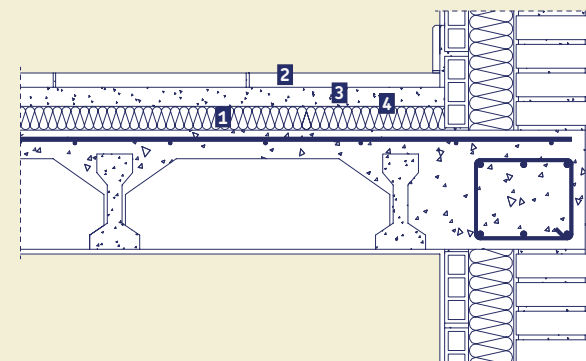
1. URSA XPS N-III I 2. Pavimento 3. Capa de compresión 4. Filtro separador
