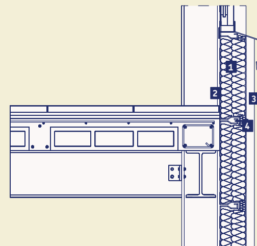
1. Doble capa URSA TERRA 2. Hoja interior de chapa 3. Hoja exterior de chapa 4. Sujeción chapa exterior
