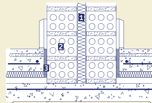
1. URSA TERRA 2. Medianera 3. Junta perimetral
