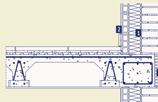
1. URSA XPS N-W E 2. Hoja interior de fábrica de ladrillo
