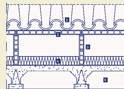
1. Teja cerámica 2. Solera de ladrillo machihembrado 3. Tabiquillo cerámico formación de pendientes con mortero 4. URSA TERRA Manta Papel 5. Forjado
