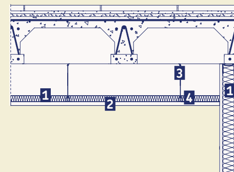
1. URSA TERRA 2. Falso techo 3. Sistema de suspensión perfiles 4. Perfil primario
