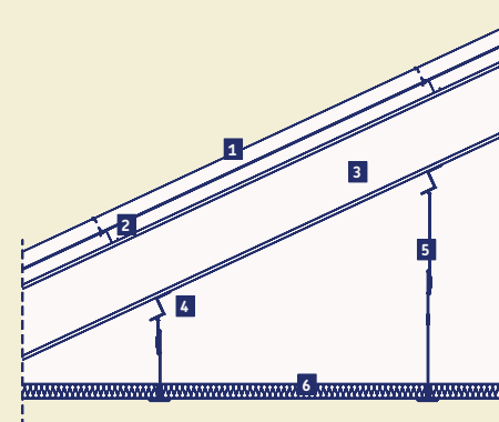
1. Cubierta chapa metálica 2. Correas metálicas 3. Estructura metálica 4. Grapa para fijación 5. Varilla roscada 6. URSA TERRA
