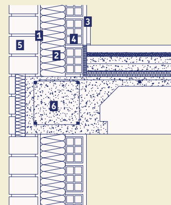
Sistema URSA MUR Detalle arranque fachada
