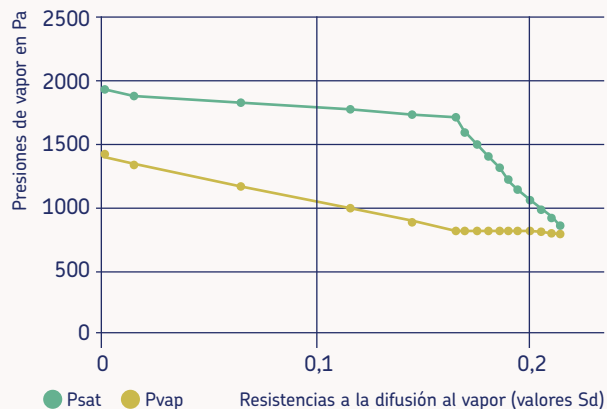
Evolución de presiones de saturación y vapor
