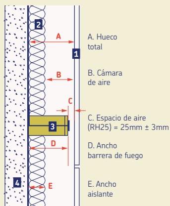
1. Revestimiento 2. URSA TERRA 3. Barrera de fuego RH 4. Muro
