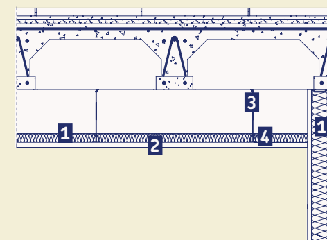
1. URSA TERRA 2. Placa perforada 3. Sistema de suspensión perfiles 4. Perfil primario
