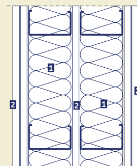
1. URSA TERRA 2. Placa yeso laminado
