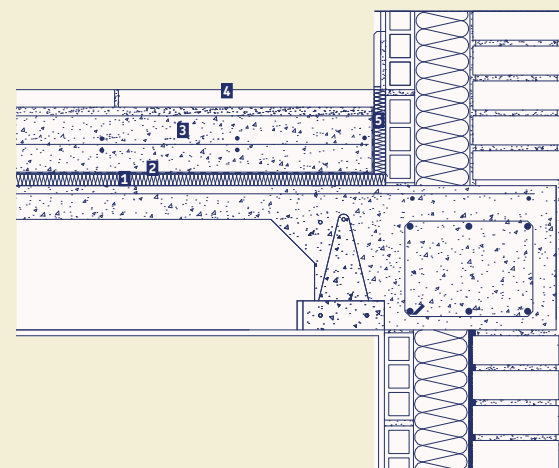
1. URSA TERRA Sol 2. Film de separación 3. Losa de hormigón armado 4. Pavimento 5. Detalles desolidarización perimetral.
