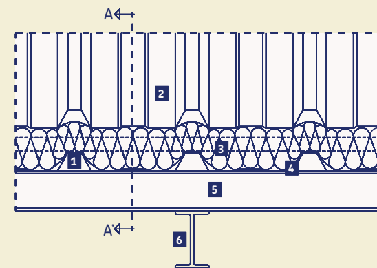
1. Omega metálica 2. Chapa metálica superior 3. URSA TERRA Manta Fieltro MNU 40 4. Chapa metálica inferior 5. Correas 6. Estructura
